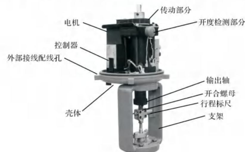
图1 执行器外观
